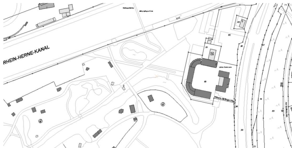
Lageplan unmaßstäblich
